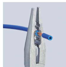
Удаление изоляции
